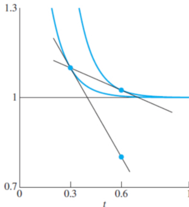
Figura 4: Comparație între pașii metodelor lui Euler și Euler implicită.
