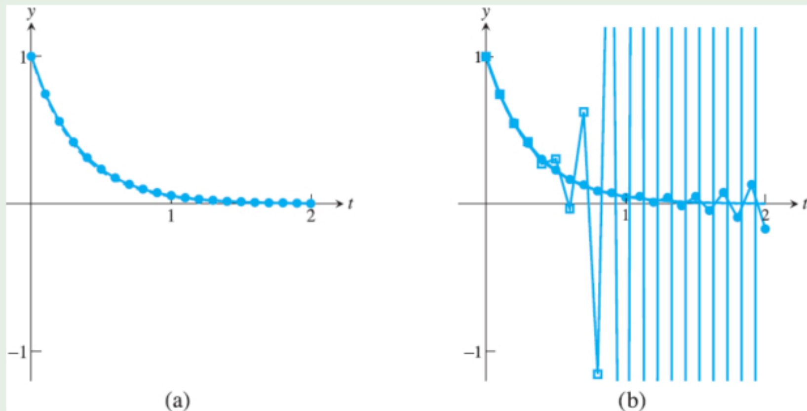
Figura 7: Comparație între metodele de ordinul doi cu doi pași aplicate PVI (41). (a) Metoda Adams–Bashforth. (b) Metoda slab stabilă (reprezentată prin puncte) și metoda instabilă (reprezentată prin pătrate).
